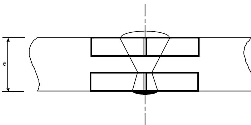
Stred zvaru
